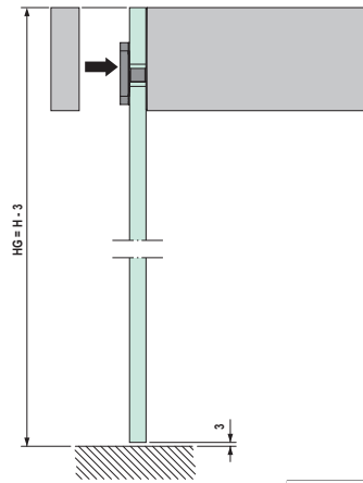
Einbausituationen mit Glaswandhalter
