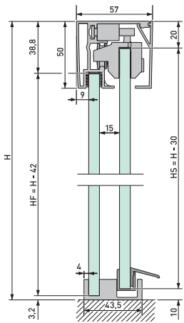
Einbausituationen mit umlaufendem Profil
