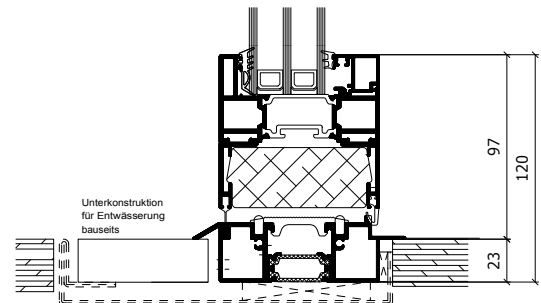
schwollenlose Ausführung
